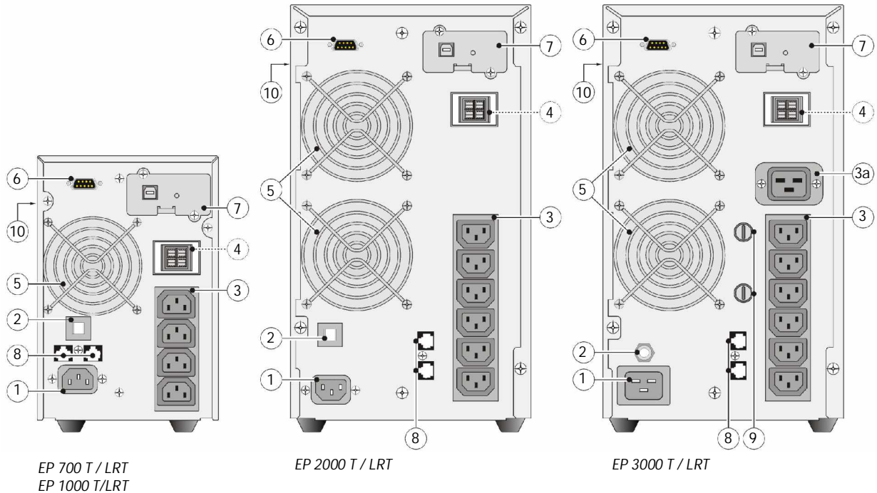
Рис. 3.3.1: задняя панель настольных моделей (EP XXXT или EP XXXLRT)
